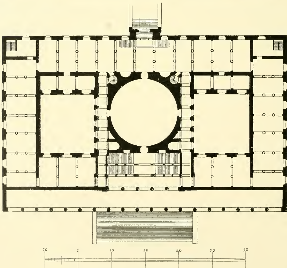
Abb. 131 Das alte Museum in Berlin Grundriß
