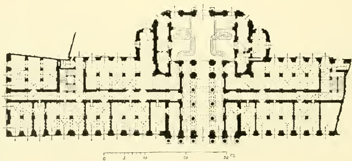
Abb. 91 Altes Landhaus in Dresden Grundriß
