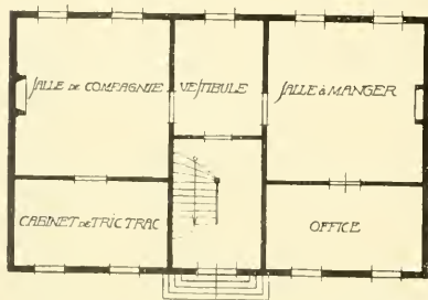
Abb. 206 Casino à l'italienne in Paris Grundriß
